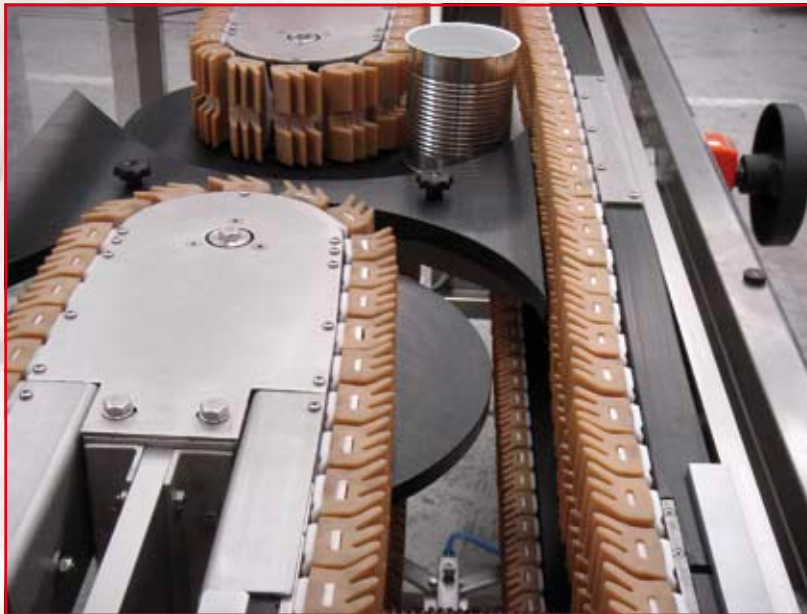
Système par pincement constitué de 2 convoyeurs parallèles
