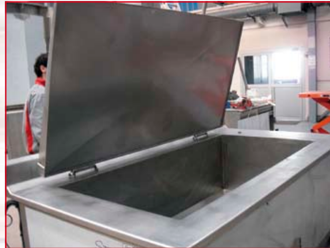
Couvercle double enveloppe assisté par charnières compensées Calorifuge 70 mm
